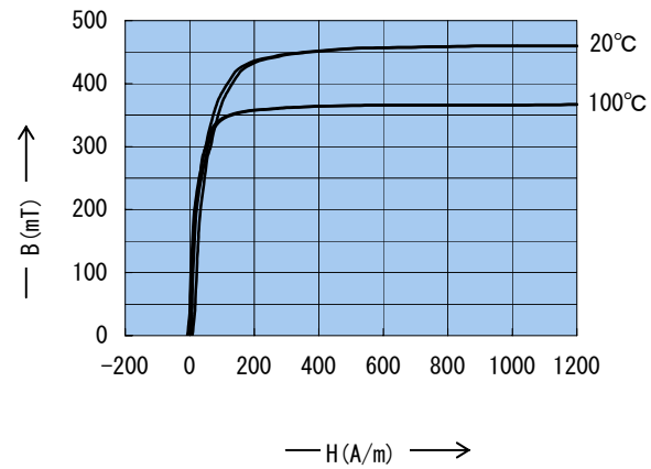
Static Magnetization Curves 直流ヒステリシス特性
