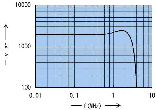
\mu_{iac} vs. Frequency \mu_{iac} 周波数特性
