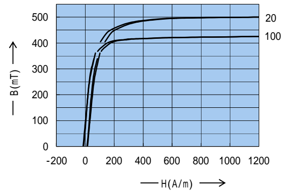
Static Magnetization Curves 直流ヒステリシス特性
