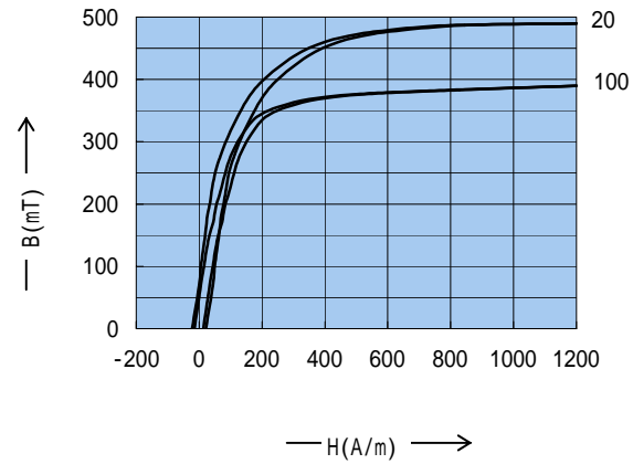
Static Magnetization Curves 直流比入特性
